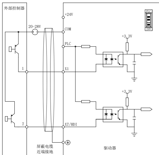
图 2-12 使用外部电源开路集电极 PNP 接线方式
