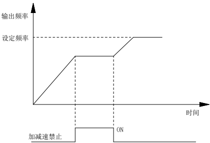
图 5-9 加减速禁止示意图
