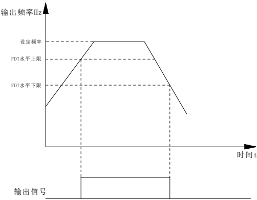
图 5-13 FDT 工作示意图
