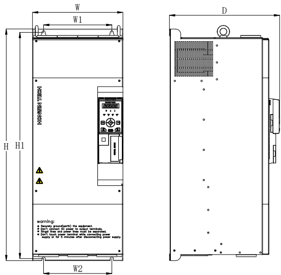
图 8-3 H150-4T18.5G~H150-4T30G 安装尺寸示意图
