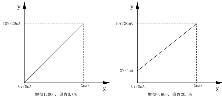
图 5-19 AO 输出示意图
