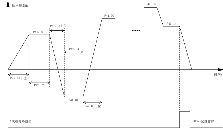
图 5-23 简易 PLC 运行示意图
