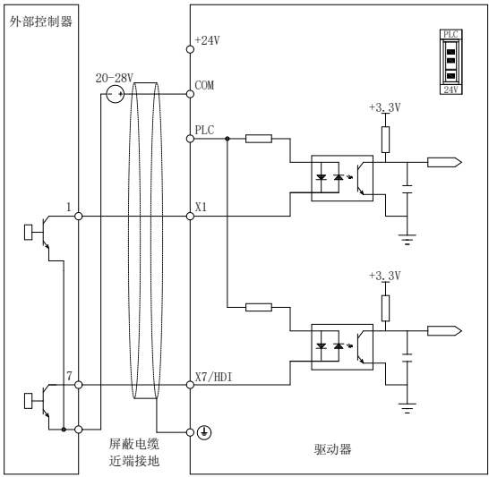
图 2-10 使用外部电源开路集电极 NPN 接线方式
