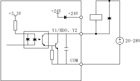
图 2-16 使用外部电源
