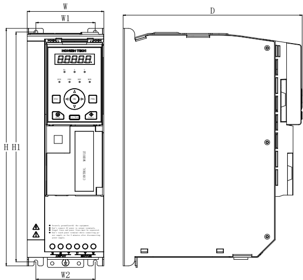
图 8-2 H150-4T7.5GB~H150-4T15GB 安装尺寸示意图
