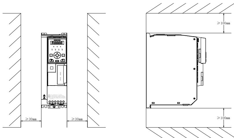
图 2-2 H150-4T15GB 及以下功率等级安装方向和空间要求
