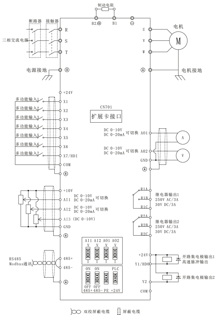
图 2-4 标准接线图
