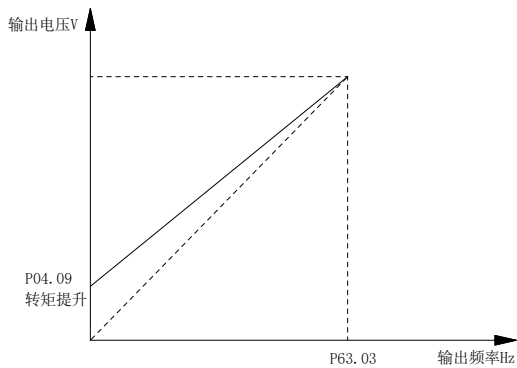
图 5-7 转矩提升示意图
