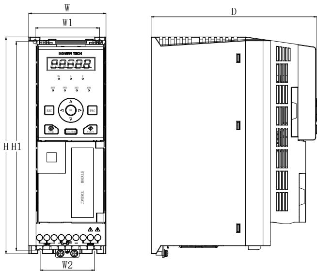
图 8-1 H150-4T5.5GB 及以下功率等级安装尺寸示意图
